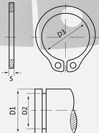
FREIOS EXTERIORES _ DIN 471
