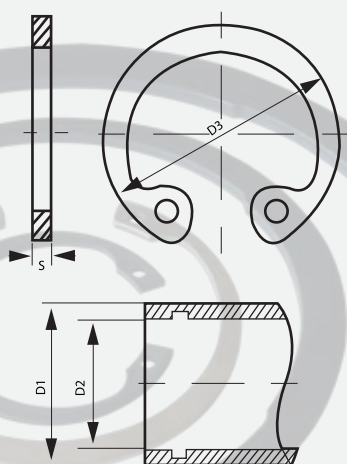
FREIOS INTERIORES _ DIN 472
