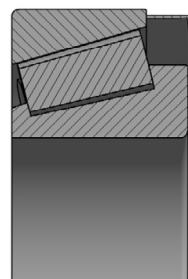
Nilo AV(3) aplicado a rolamentos de rolos cônicos em polegadas
