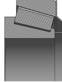
Nilo JV(2) aplicado a rolamentos de rolos cônicos com anel interior mais baixo
