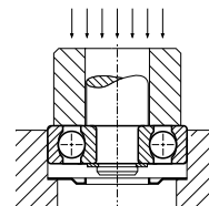
Método correto de montagem do veio em rolamentos de esferas.
