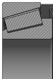
Nilo AV(2) aplicado a rolamentos de rolos
