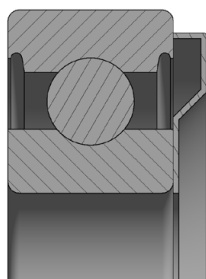
Nilo AV(1) aplicado a rolamentos de esferas
