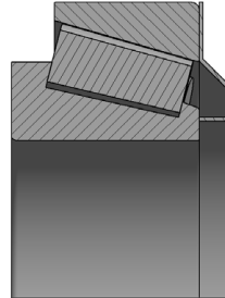
Nilo JV(1) aplicado a rolamentos de rolos cônicos com anel interior à face
