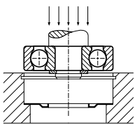
Método incorreto de montagem do veio no rolamento de esferas sem a utilização de um auxiliar de montagem.
