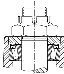
17.4 - Montagem final no Nilo AK
