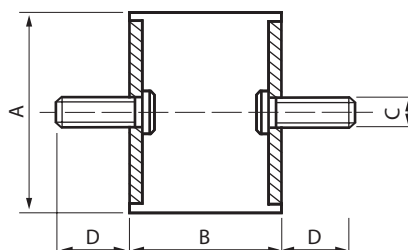
a) A - Diâmetro exterior do Apoio | B - Altura | C - Diâmetro do Perne | D - Comprimento do Perne
