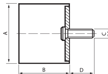
a) A - Diâmetro exterior do Apoio | B - Altura | C - Diâmetro do Perne | D - Comprimento do Perne
