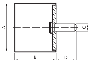
a) A - Diâmetro exterior do Apoio | B - Altura | C - Diâmetro do Perne | D - Comprimento do Perne
